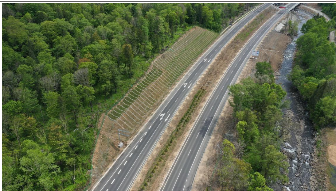
龙蒲 4 标 K89+000 主线路基挖填方边坡，挖方边坡坡面实施叠拱防护，坡脚边沟，坡面实施灌草绿化，填方边坡坡脚边沟，坡面实施灌草绿化，中央分隔带实施灌木栽植、植草绿化托植物措施。
